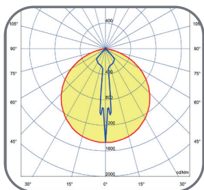
CURVA FOTOMÉTRICA LED-HB 5212-FC EXTREME
