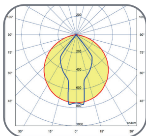
CURVA FOTOMÉTRICA LED-HB 5212-FM EXTREME
